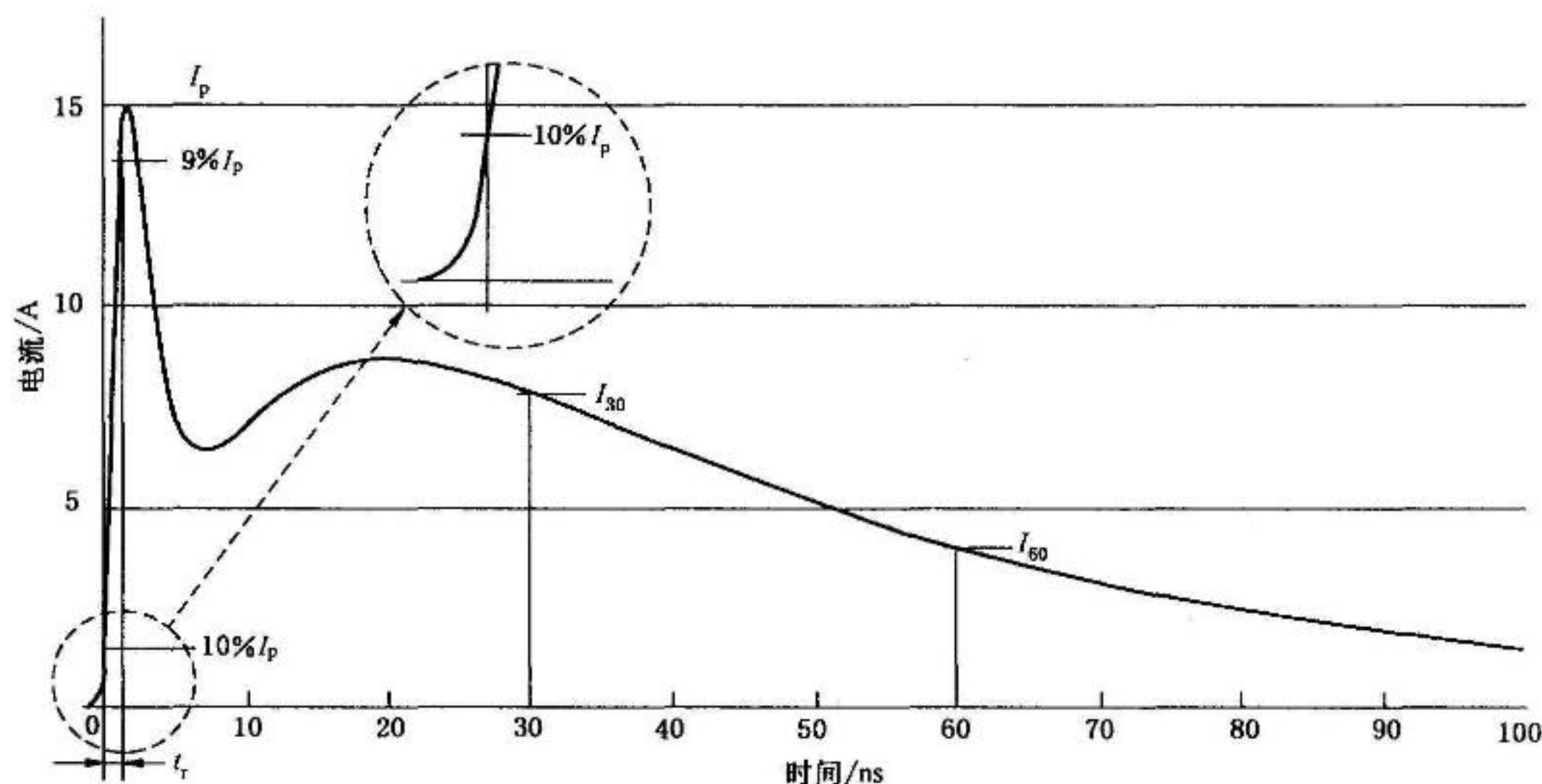
图2 接触放电电流波形
