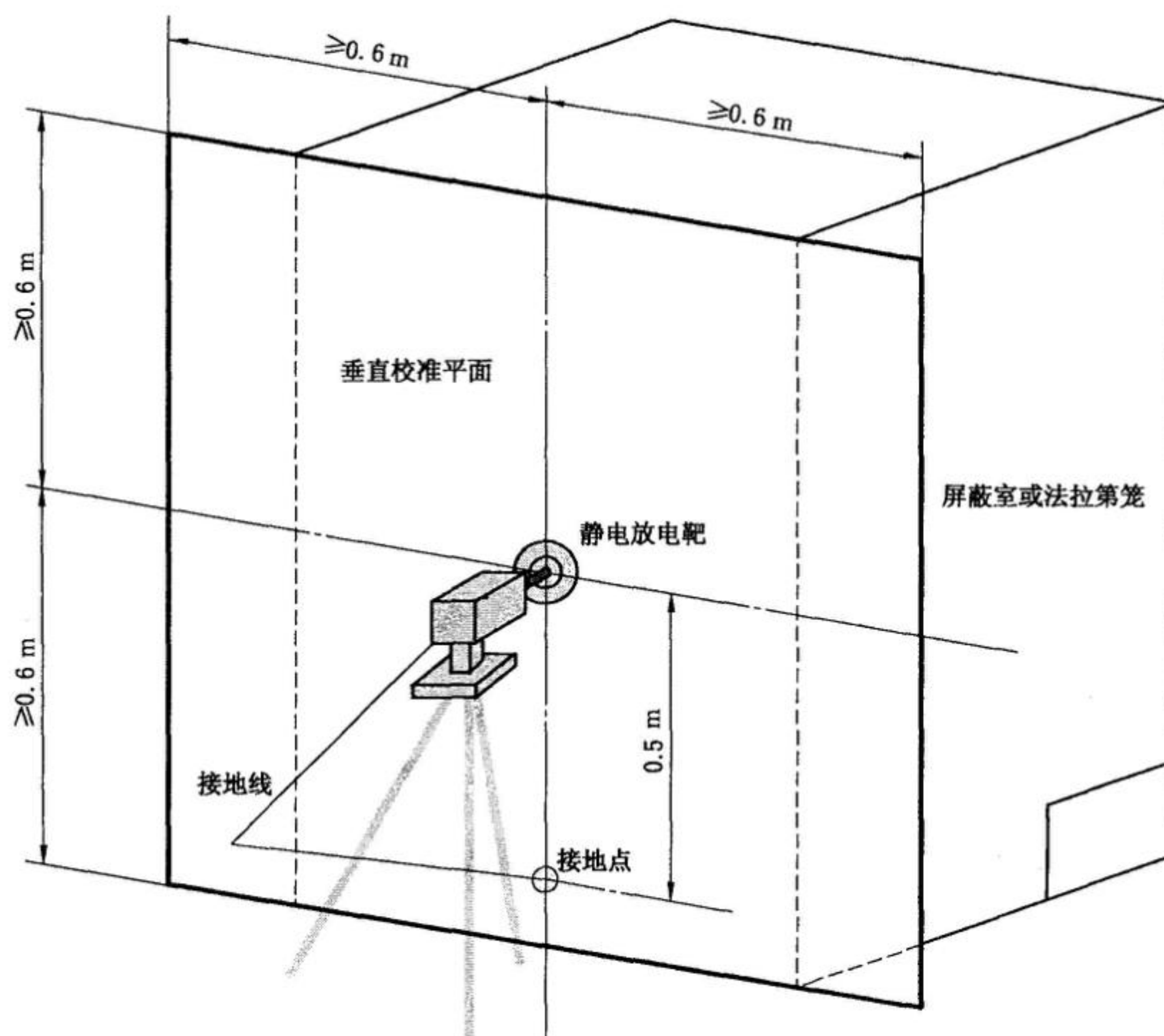
图4 静电放电模拟器校准连接示意图
